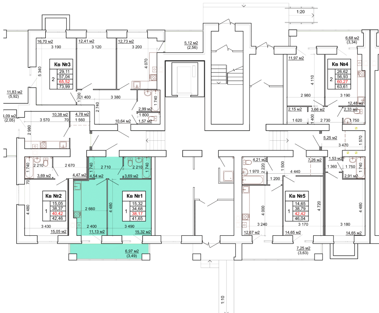
План 1-го этажа Секция в осях 1-2
